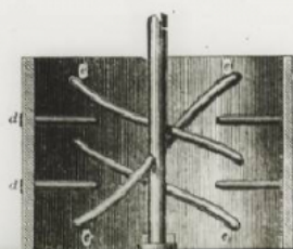
Malaxeur de machine précédente.
