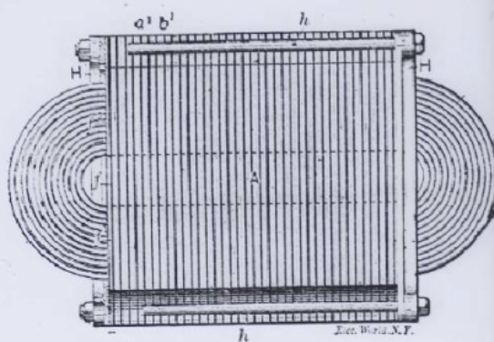
— Transformateur Westinghouse.
