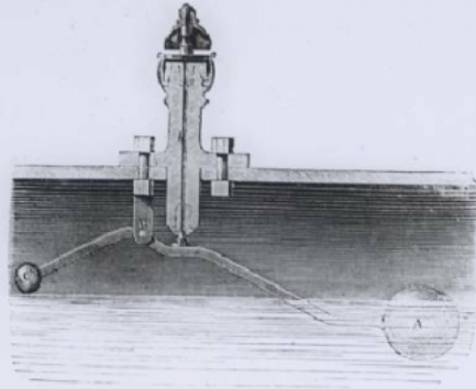
— Flotteur Sifflet d'alarme.
