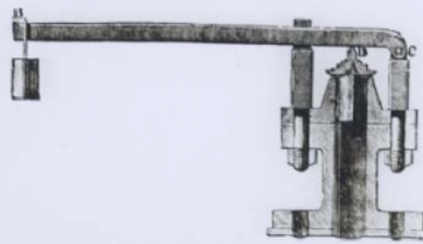
— Soupape de sûreté.
