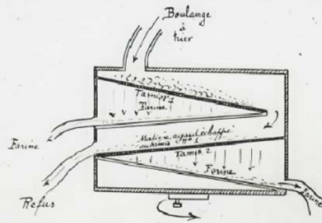
Principe du plansichter
