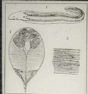
Organes electriques du gymnote. — 1. Vue d'ensemble de l'organe. — 2. Coupe d'un gymnote. — 3. Vue au microscope des cellules de l'organe.
