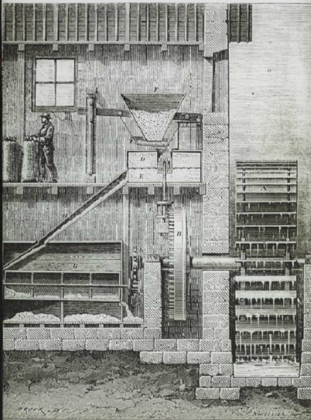
Fig. 13. — Le moulin à eau appliqué à la mouture du blé (coupes verticales).
