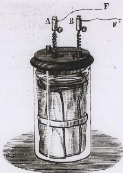
Élément de pile secondaire.
