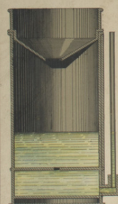
PLUVIOMÈTRE (Coupe) Appareil destiné à mesurer la quantité d'eau de pluie tombée en un lieu.
