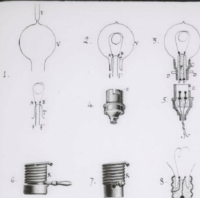
Fabrication d'une Lampe à incandescence Doutilles et Cutois.
