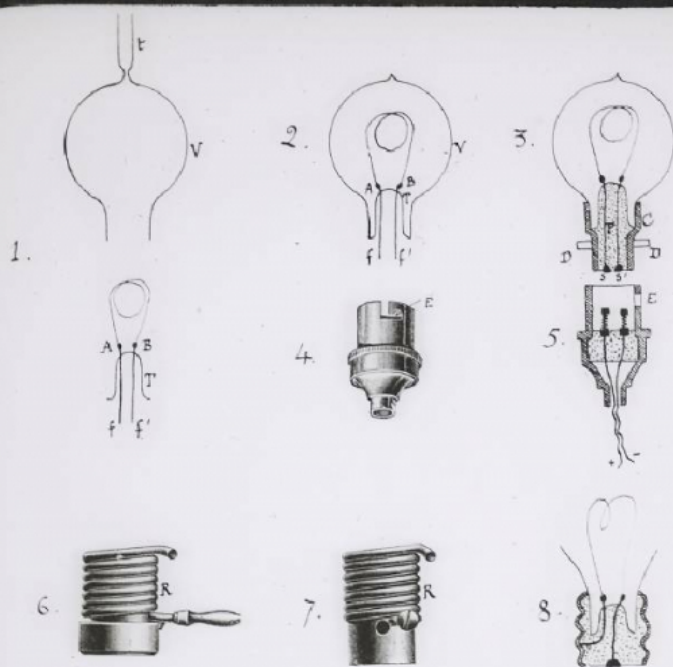
Fabrication d'une Lampe à incandescence Détails et Cutois.
