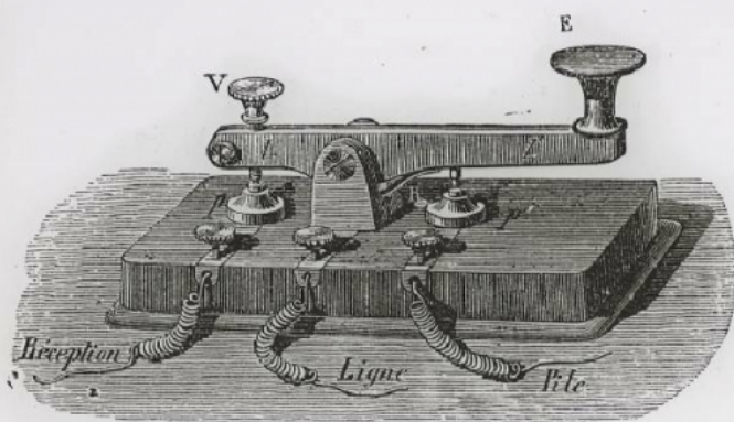
- Manipulateur de l'appareil Morse à pointe sèche.
