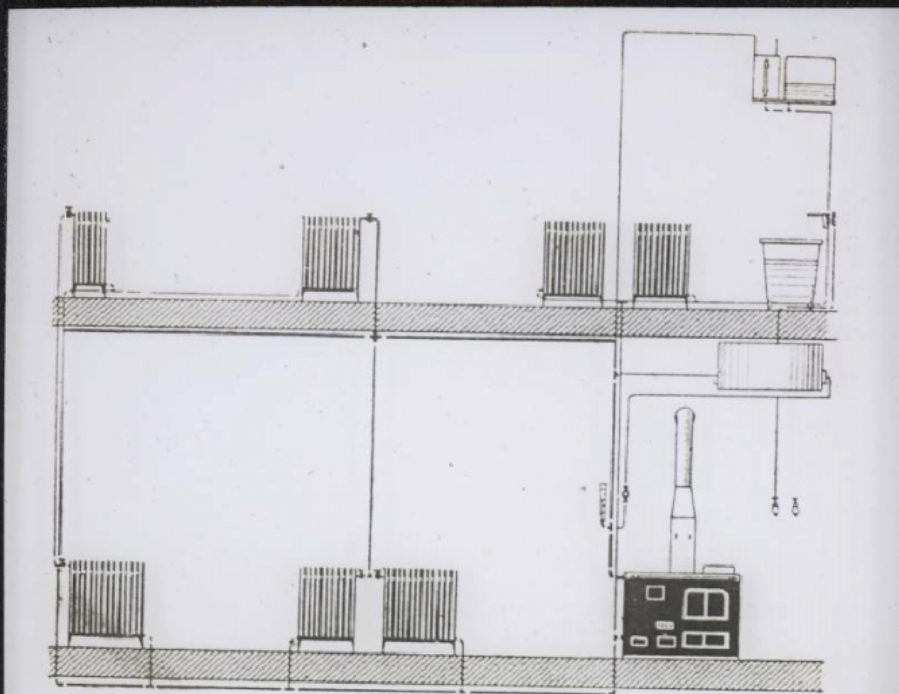
Schéma d'installation de chauffage central, la cuisine servant de foyer.
