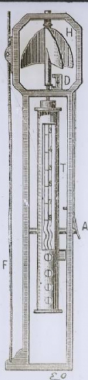
Appareil à retournement de l'amiral Magnaghi.
