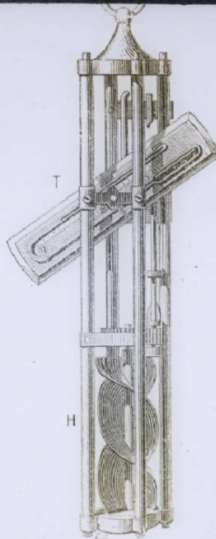
Fig. 139. — Dispositif destiné à produire le retournement d'un thermomètre Segretti.
