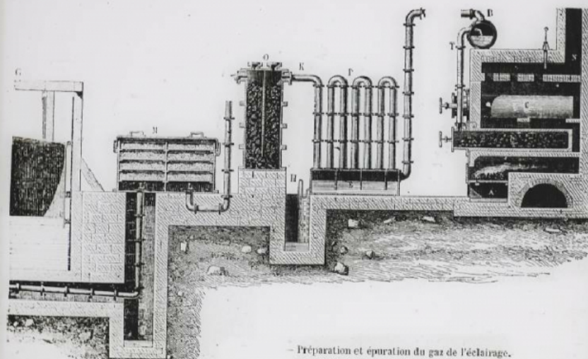
- Préparation et épuration du gaz de l'éclairage.
