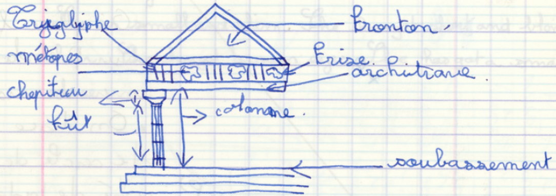
Ordre dorique.
