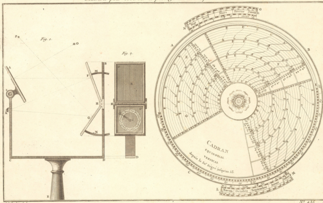
Machine pour observer le passage des Astres par le Méridien.
